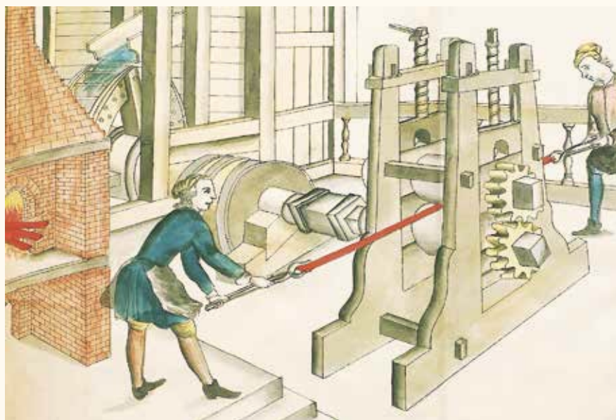
Плющильная машина. Рисунок из книги В. И. Геннина «Описание Уральских и Сибирских заводов»
