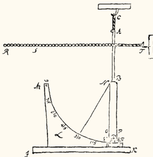
Электрический указатель, применявшийся при исследовании грозы. Рисунок Рихмана
