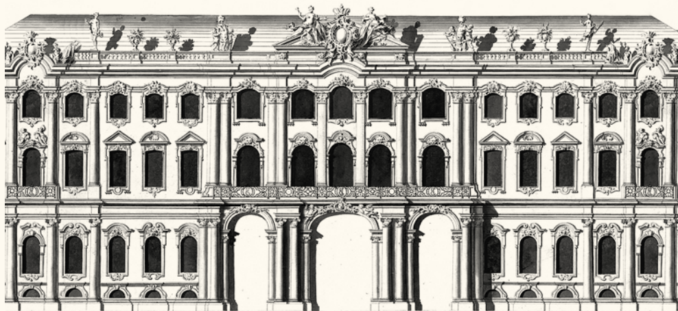
Авторский проект фасада Зимнего дворца. Фрагмент
